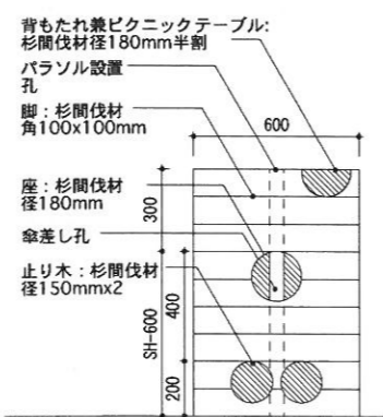
SH-600タイプ断面図 s.1/30
