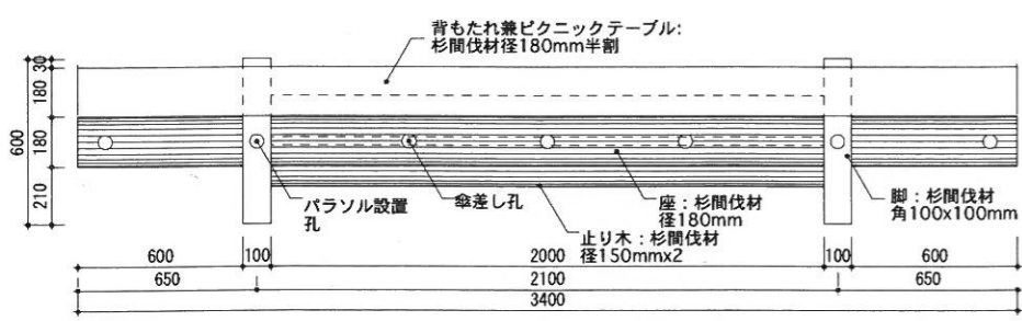
SH-600タイプ平面図 s.1/30
