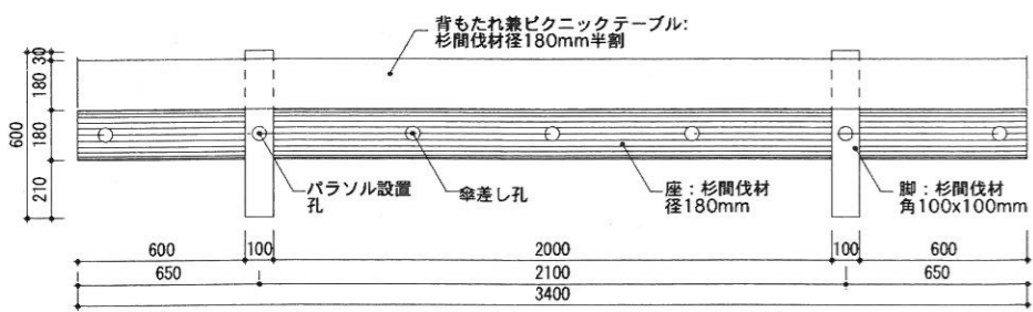
SH-400タイプ平面図 s.1/30
