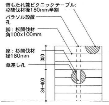
SH-400タイプ断面図 s.1/30
