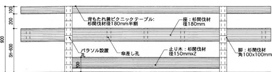
SH-600タイプ立面図 s.1/30
