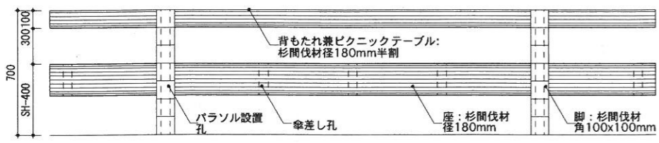
SH-400タイプ立面図 s.1/30
